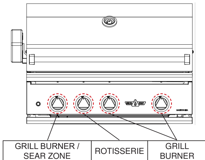
DHBQ32R/S-D
